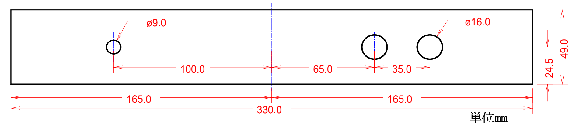
図35 モーター制御部フロントパネル
