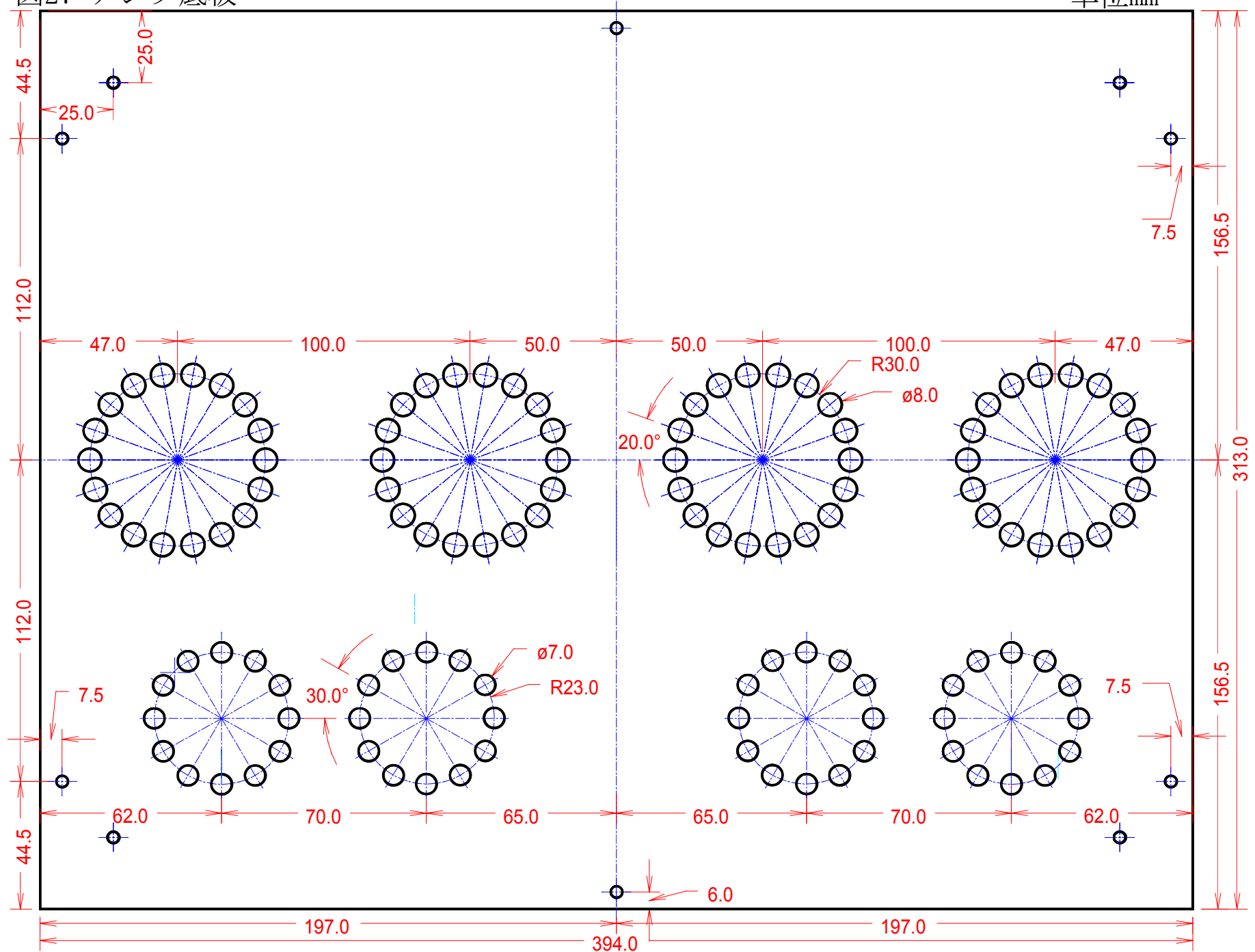
図27 アンプ底板
