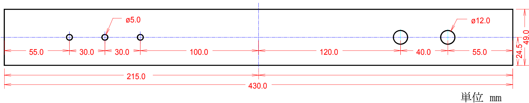
図24 フロントパネル
